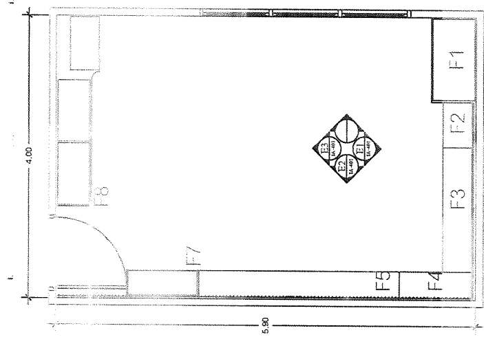
แปลนห้องสำนักงาน 1:100 (ค.พ.ก.)
